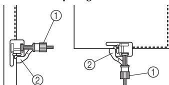
① Tornillo ② Guía
