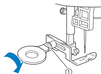
① Fixierschraube
