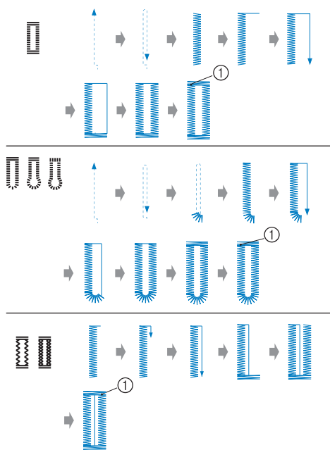
① Verstärkungsstiche
