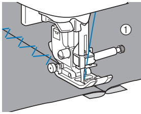
① Stoffvorderseite
