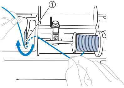
① Fadenführungsplatte
