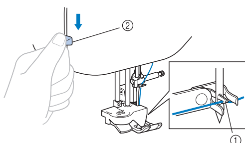
① Haken ② Nadeleinfädlerhebel
