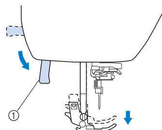
① Levier du pied-de-biche
