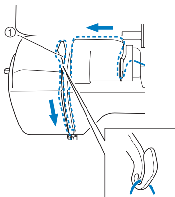
① Levier releveur
