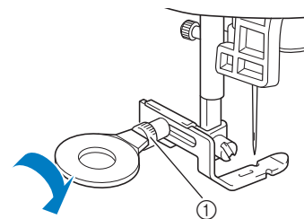
① Vis de positionnement
