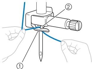
① Guida del filo della barra dell'ago ② Linguetta
