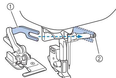
① Forcella di collegamento ② Vite morsetto ago
