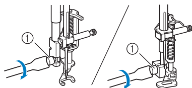
① Vite del supporto del piedino premistoffa
