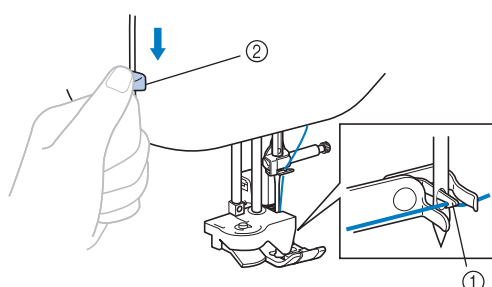
① Uncino ② Leva dell'infilago
