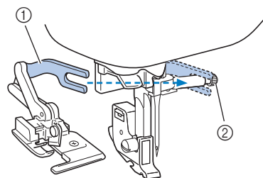
① Horca de conexión ② Tornillo de la presilla de la aguja
