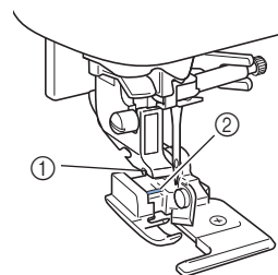
① Muesca del soporte del pie prensatela ② Patilla
