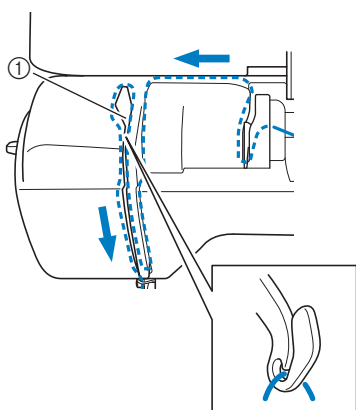
① Levier releveur
