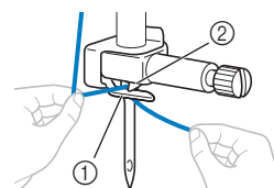
① Fadenführung an der Nadelstange ② Lasche
