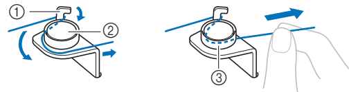
① Draadgeleider voor het opwinden van de spoel ② Voorspanning voor spoelen ③ Trek de draad zo ver mogelijk naar binnen.
