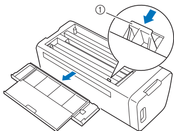
① Palanca de liberación de la bandeja posterior
