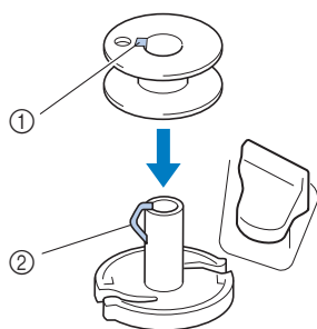
① Rainure de la canette ② Ressort de l'axe
