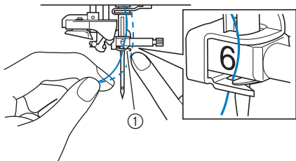
① Guide-fil de la barre de l'aiguille
