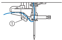
① Rainure du guide-fil
