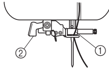
① 针杆 ② 穿线器拨杆
