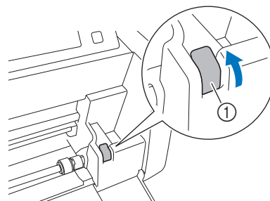
① Ontgrendelingshendel voor transporteur
