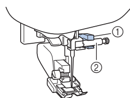
① ふたまた部 ② 針のとめネジ
