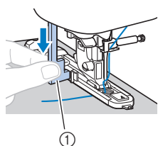
① ボタン穴かがりレバー
