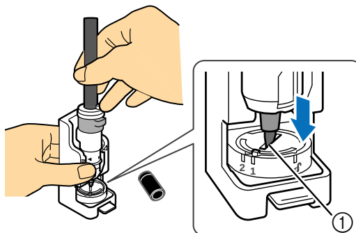
① Nut
