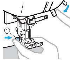
(1) Baskı ayağı tutma iğnesi
