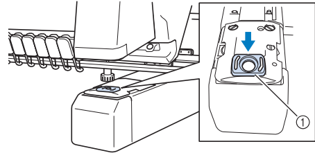
① Capot de la plaque à aiguille
