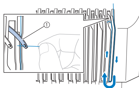
① Levier releveur de fils
