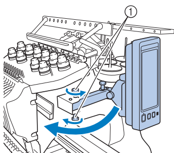
① Vis de serrage à main
