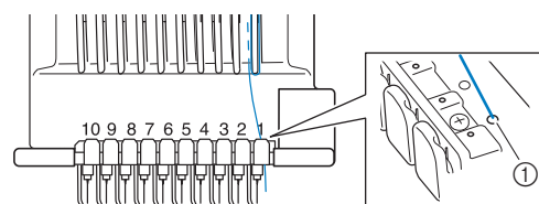
① Trou du guide-fil inférieur
