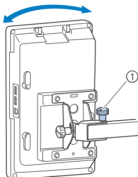
① Vis de serrage à main
