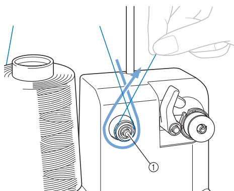
① Disque de tension
