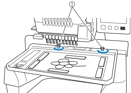
① Vis de serrage à main
