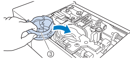
① Marque ▲ sur le boîtier de canette ② Marque ● sur la machine ③ Boîtier de canette
