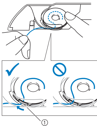
① Ressort de tension
