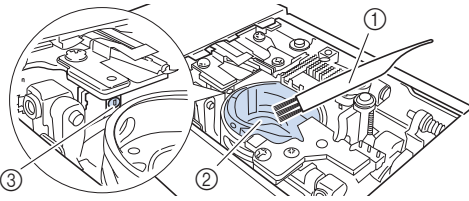
① Brosse de nettoyage ② Coursière ③ Capteur de fil de canette
