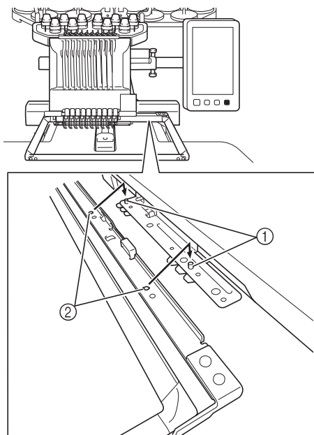
① X キャリッジのピン ② マグネット原反枠の穴
