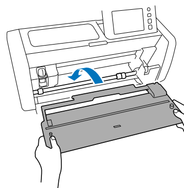
① Levier de déverrouillage du système d'entraînement ► Seul le côté droit de l'axe se baisse, et l'axe se verrouille.
