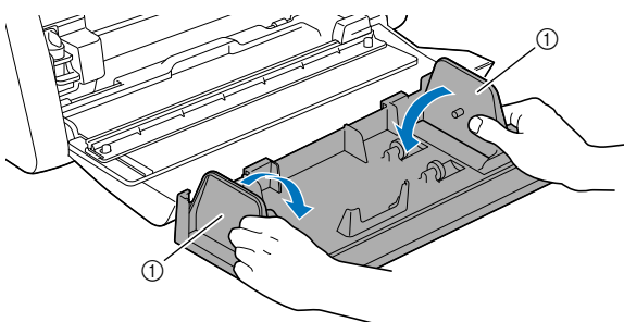
① Geleiderplaat
