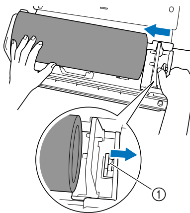
① Afstelhendel
