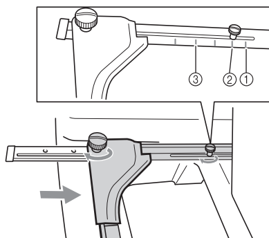
① ジャンボ枠のマーク 360mm × 360mm ② ボーダー枠のマーク 100mm × 300mm ③ キルト枠のマーク 200mm × 200mm
