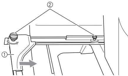
① 원팔 ② 손잡이 나사
