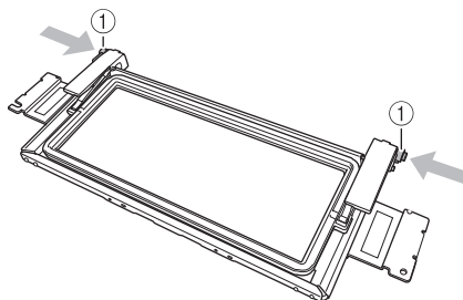
① ロック解除ボタン
