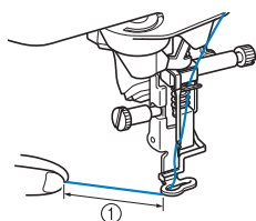
① Environ 10 cm (env. 4" / pouces)
