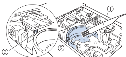
① Brosse de nettoyage ② Coursière ③ Capteur de fil de la canette
