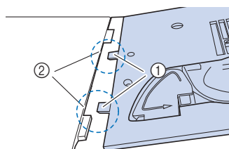
① Taquets ② Encoches
