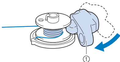
① Spoelopwindschakelaar
