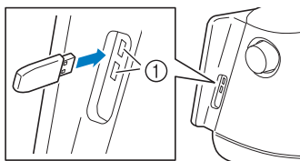
① USB-poorten
