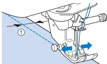
① L/R-versc.
