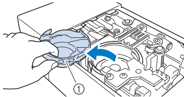
① Spoelhuis
