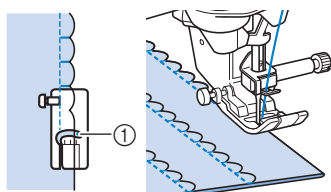
① 針落ち位置
