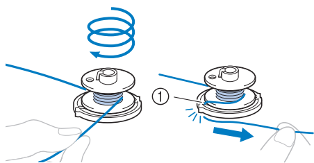
① ガイドミゾ (カッター付)
