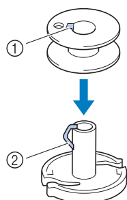
① ボピンのミゾ ② 下糸巻き軸のバネ
