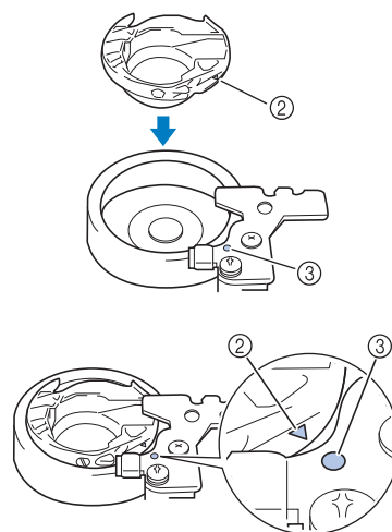
① 内かま ② 内かまの▲印 ③ ミシンの●印
