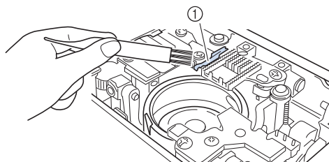
① カッター
