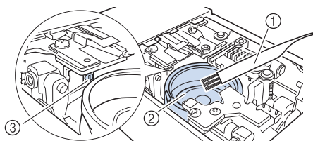
① ミシンブラシ ② 外かま ③ 下糸センサー
