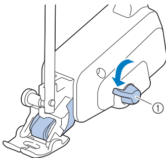
① フィード位置レバー
