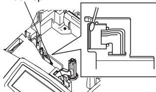
Druckkopf
