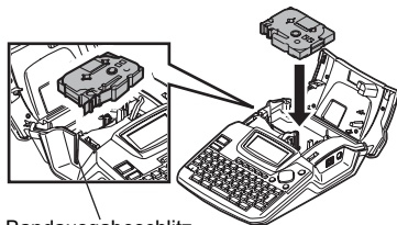
Bandausgabeschlitz
