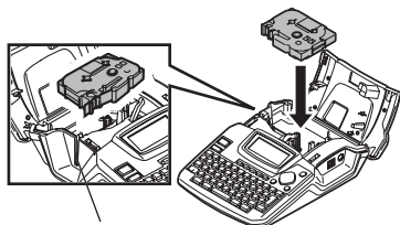
Fessura di uscita del nastro
