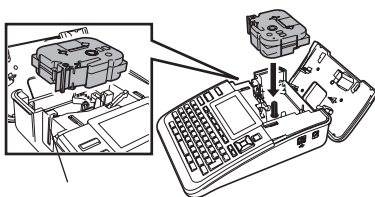
Ranhura de saída da fita
