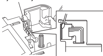
Nyomtatófej
