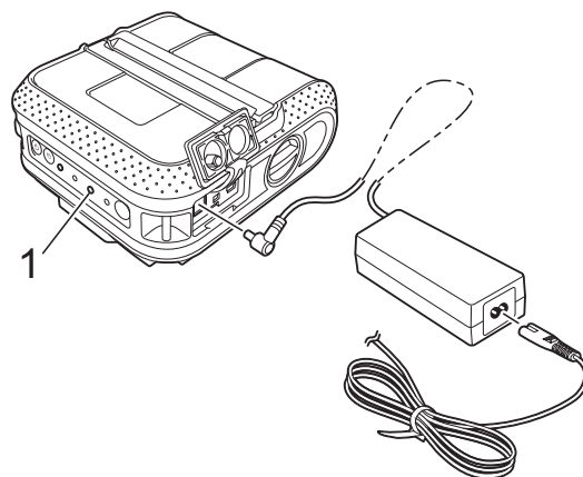
1 Indicador BATT (batería)
