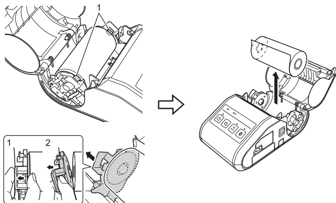
1 Rullefrigørelseshåndtag
