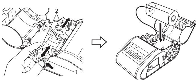
1 Rolleneinstellungshebel 2 Rollenführung
