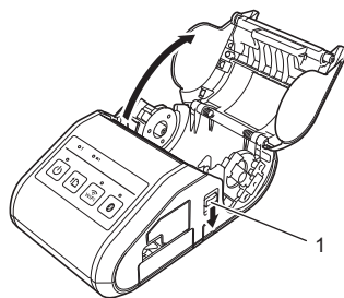
1 Hebel zum Öffnen der Abdeckung
