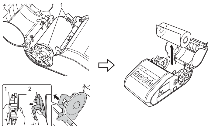
1 Hebel für die Rollenfreigabe
