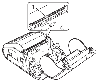
1 Druckkopf
