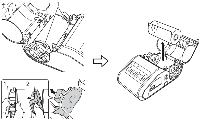
1 Rullens frigöringsspak
