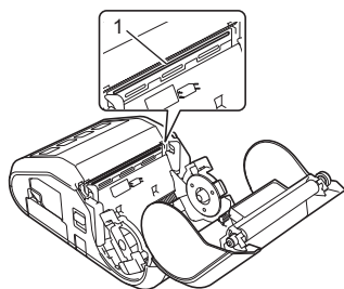
1 Skrivhuvud
