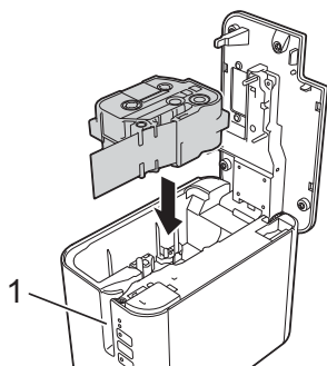
1 Tapeutgangens åpning
