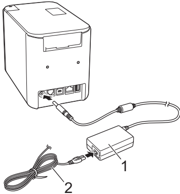
1 Nettadapter 2 Strømledning
