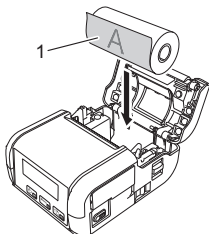
1 Superficie de impresión (cara externa del rollo)
