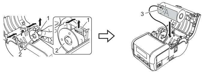
1 Palanca de ajuste de la guía del rollo 2 Guía del rollo 3 Superficie de impresión (cara externa del rollo)
