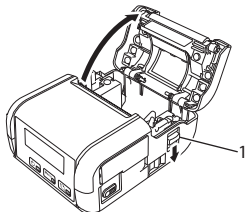
1 Palanca de apertura de la cubierta
