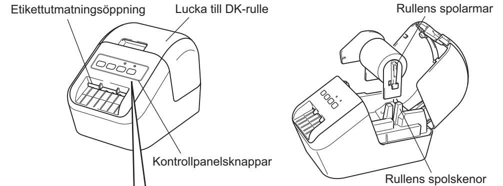
Kontrollpanelsknappar
