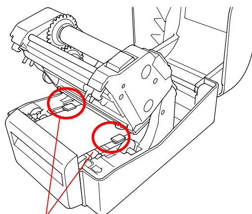
Embouts des guides de support
