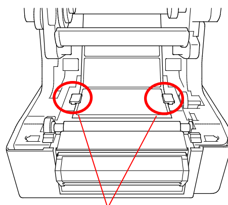
Embouts des guides de support
