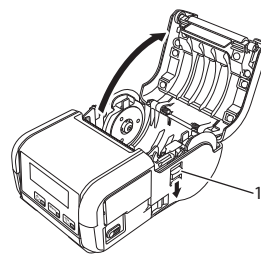
1 Kannen avaamisvipu
